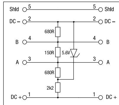
Стабилизатор сети PK6 со встроенным сопротивлением нагрузки.
